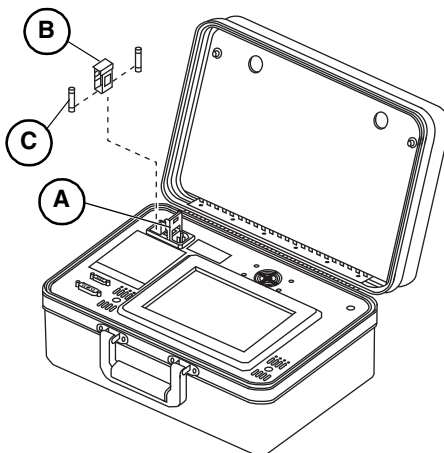
Figura 70 – Sustitución de fusibles
