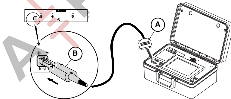
Figura 2 – Conexión a las unidades de disparo STR
