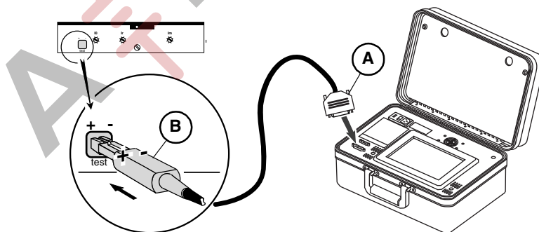
Figure 2 – Raccordement aux déclencheurs STR
